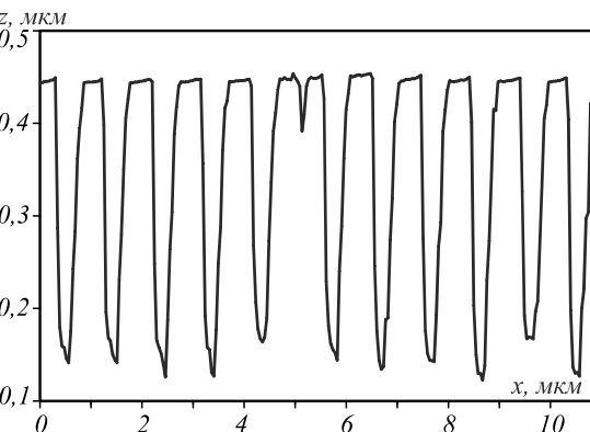
Рис. 5. Рельеф изготовленного ВА с m = 2 (а) и его сечение вдоль оси y (б), измеренные на атомно-силовом микроскопе
