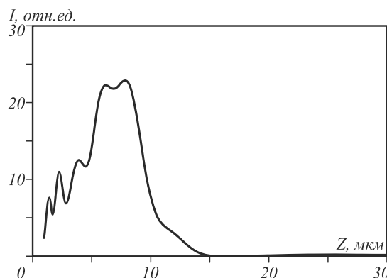
Рис. 3. Зависимость интенсивности на оси от расстояния z для аксикона с m=0
