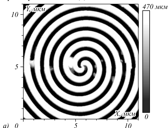
Рис. 5. Рельеф изготовленного ВА с m = 2 (а) и его сечение вдоль оси y (б), измеренные на атомно-силовом микроскопе
